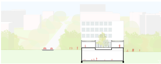
Schnitt A - A
